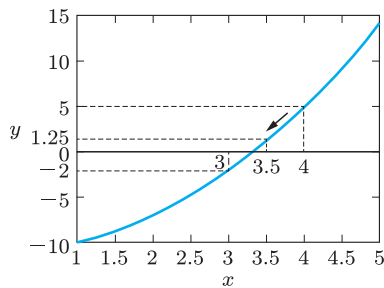
(b) 第2近似根は3.5
