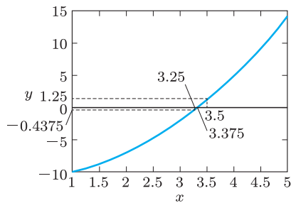
(d) 第4近似根は3.375 (第5近似根は3.3125)
