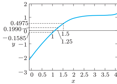
(d) 第4近似根は1.25
