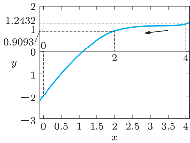
(a) 第1近似根は2
