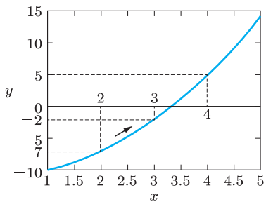
(a) 第1近似根は3
