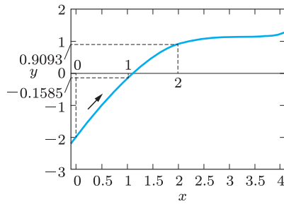
(b) 第2近似根は1
