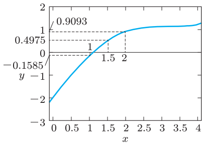
(c) 第3近似根は1.5
