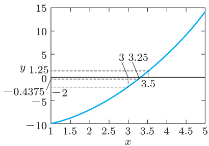
(c) 第3近似根は3.25
