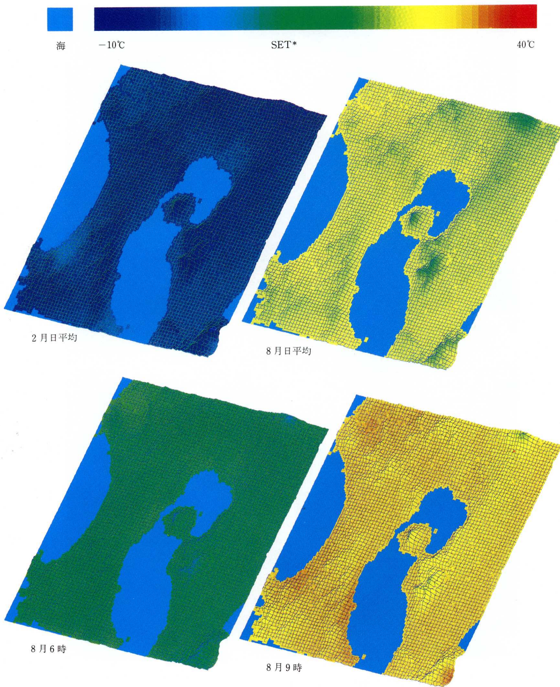
図 2.10 標準新有効温度 (SET*) のマップの例 (鹿児島県) (高さは約 2 倍に強調, ワイヤーの間隔は約 1 km) (その 1)
